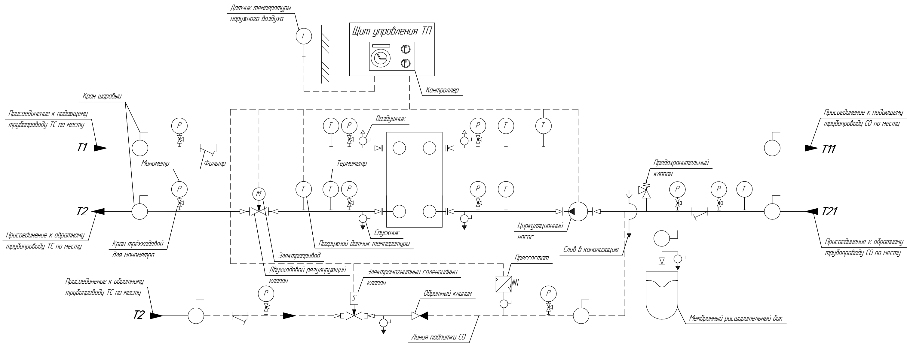
Схема обвязки ПТО для независимой системы отопления
